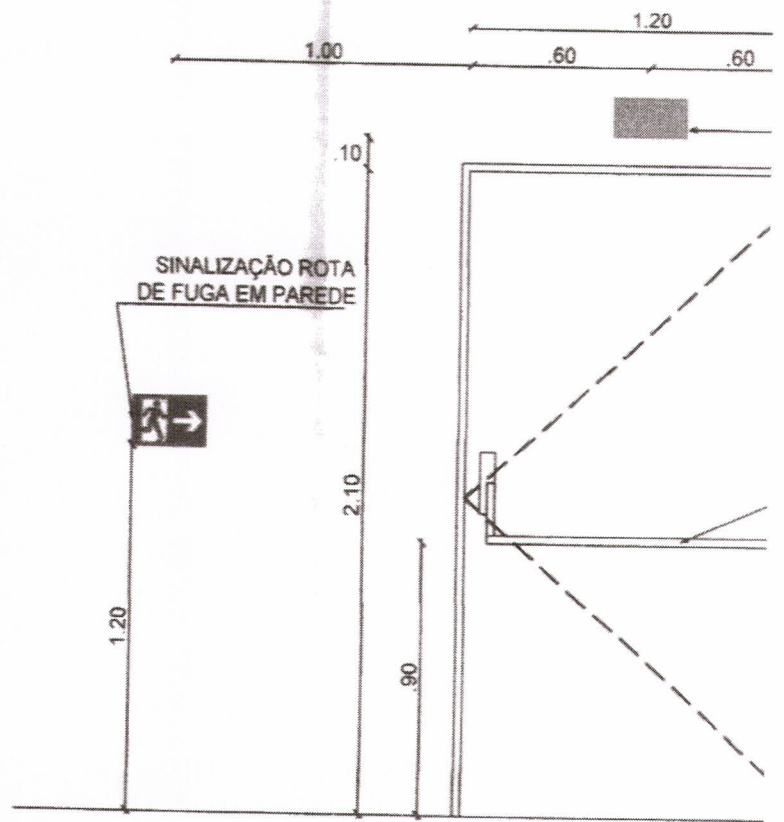
2 DETALHE SAÍDA DE EMERGÊNC ESCALA 1:25
