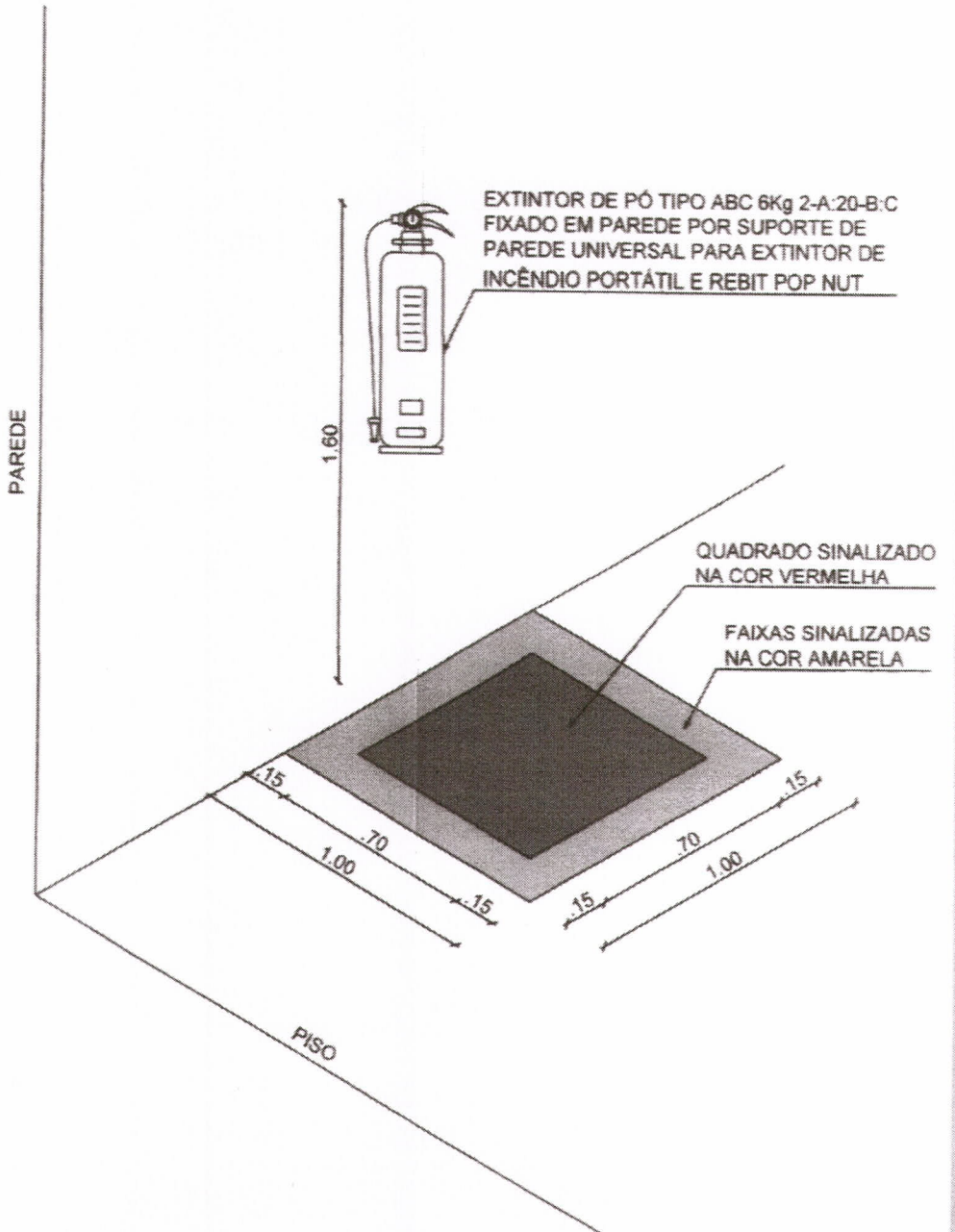
3 DETALHE ISOMÉTRICO - EXTINTOR E MARCAÇÃO NO PISO ESCALA 1:25
