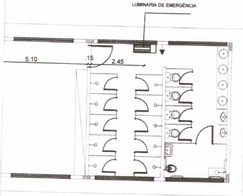
1 PLANTA DE INCÊNDIO E SINALIZAÇÃO DE EMERGÊNCIA ESCALA 1:100
